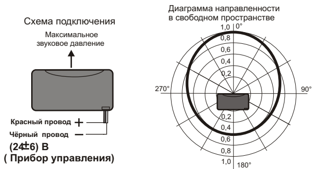
Рис.2 Схема подключения и диаграмма направленности звука оповещателя.
