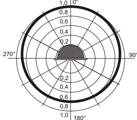
Диаграмма направленности в свободном пространстве
