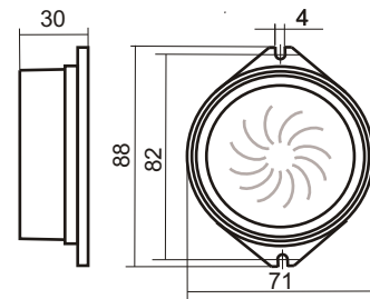
Рис.1. Габаритные и установочные размеры
