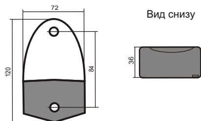
Рис.1. Габаритные и установочные размеры оповещателя
